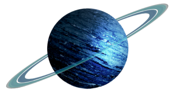
Uranus
