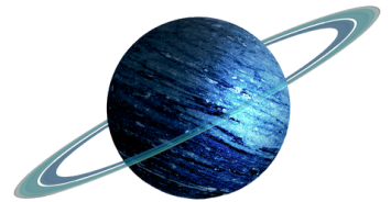
Uranus
